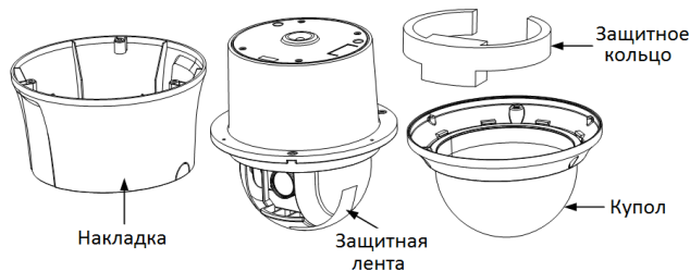
Рисунок 1-11 Демонтаж камеры
